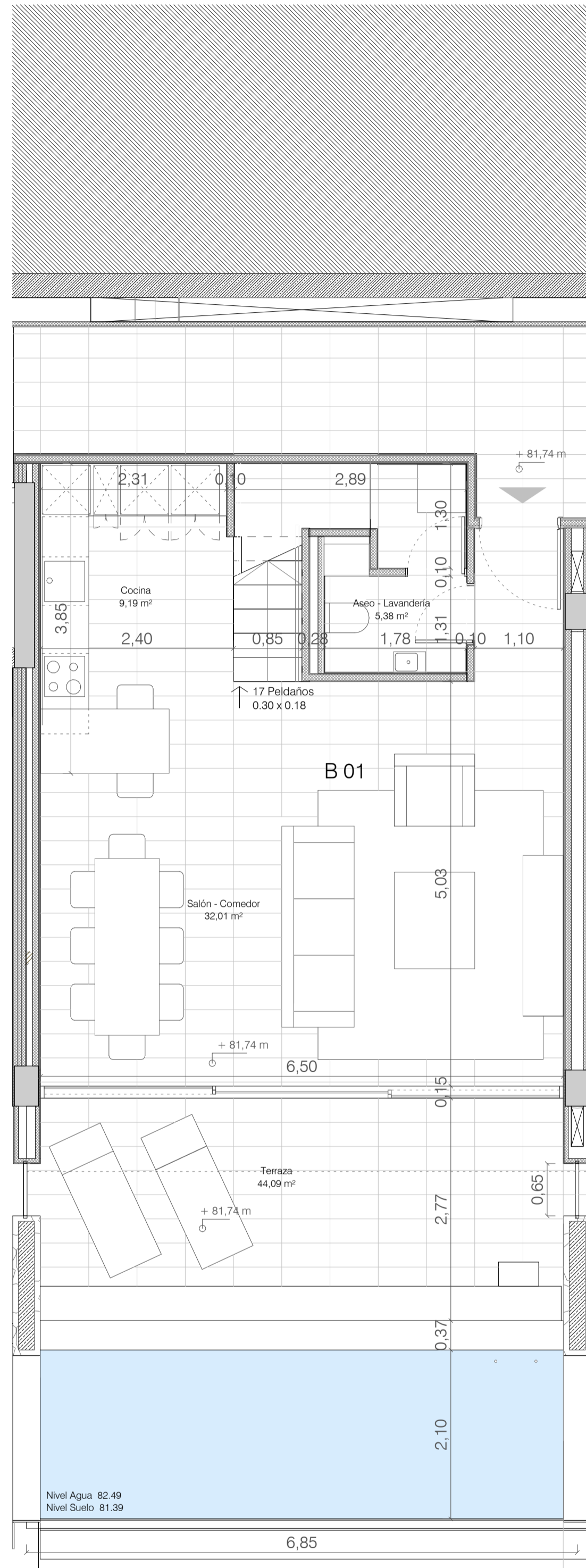
B01_P_Baja A1 e - 1 : 50
