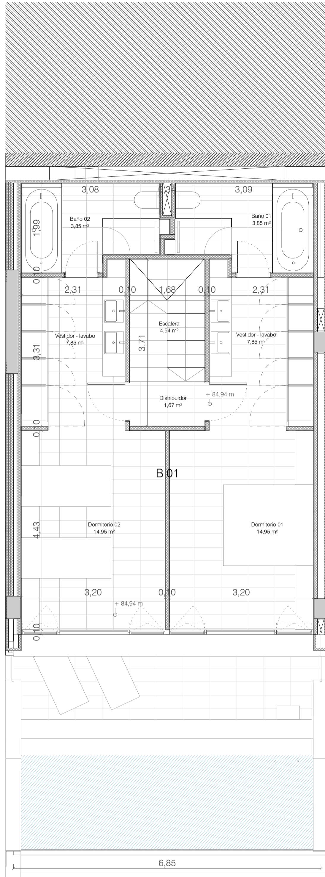
B01_P_Alta A1 e - 1 : 50
